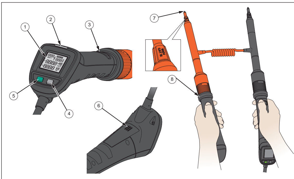
Afbeelding 4-1. BTL20 Interactive Test Probe
