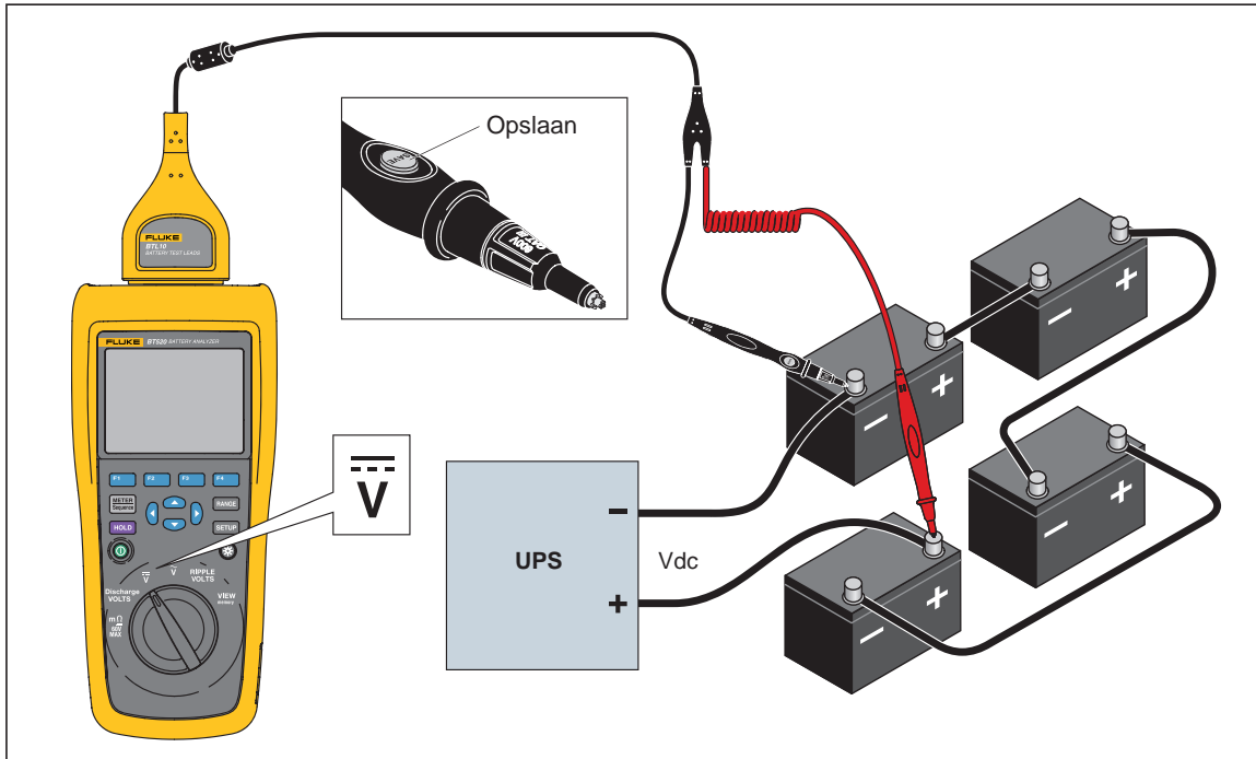
Afbeelding 3-3. DC-spanning meten
