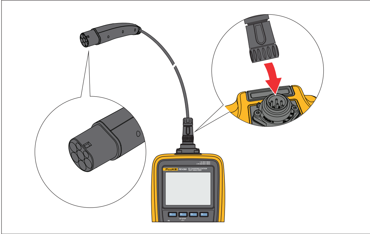
Afbeelding 1. De stekker aansluiten
